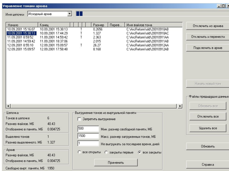
Рисунок 14 Окно Управление томами архива
