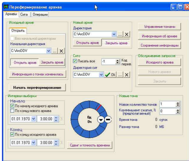
Рисунок 6 - Окно закладки Архивы
