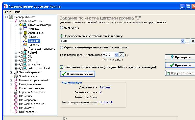
Рисунок 26 - Ход выполнения операции.
