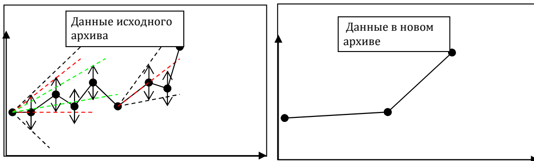
Рисунок 19 - Линейная апертура
