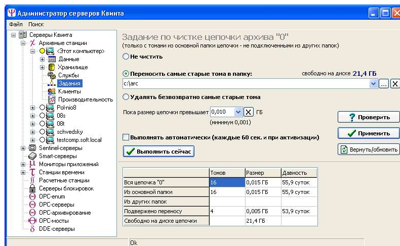
Рисунок 25 - Окно для формирования задания.
