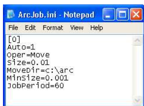
Рисунок 28 - ini-файл, в котором хранится настройка операции
