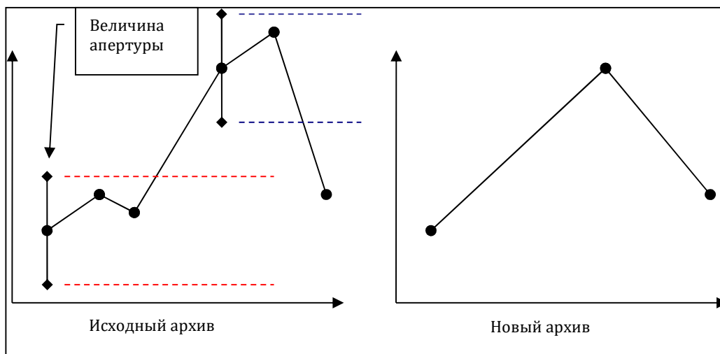
Рисунок 18 - Нелинейная апертура
