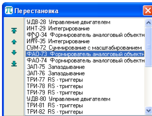
Рисунок 28 - Диалоговое окно перестановки алгоблоков
