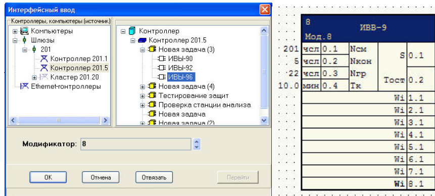
Рисунок 24 - Установка уникальной константы (пример 2б)
