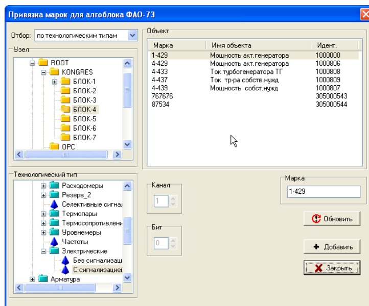
Рисунок 31 - Выбор объекта привязки
