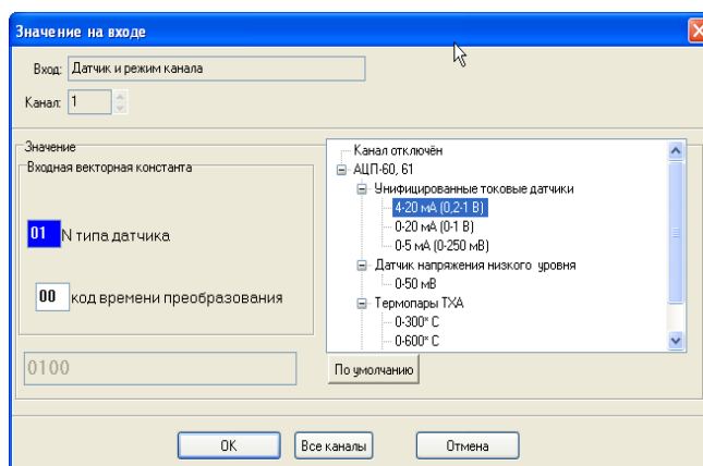
Рисунок 21 - Выбор параметров на векторном входе (пример)
