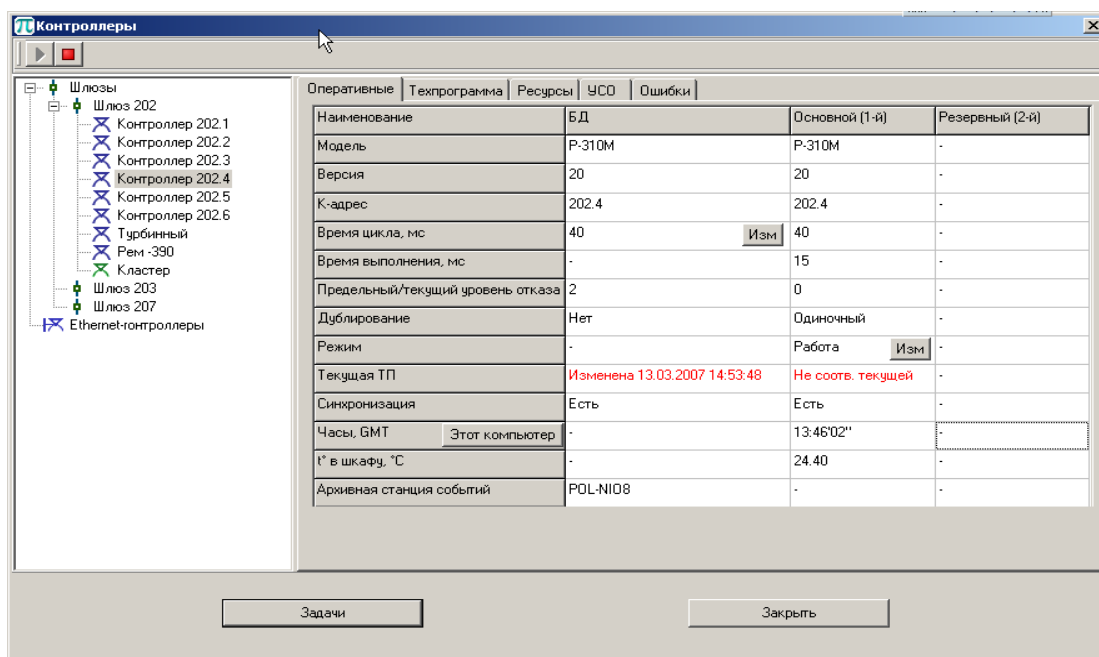
Рисунок 2 - Окно Контроллеры. Закладка Оперативные
