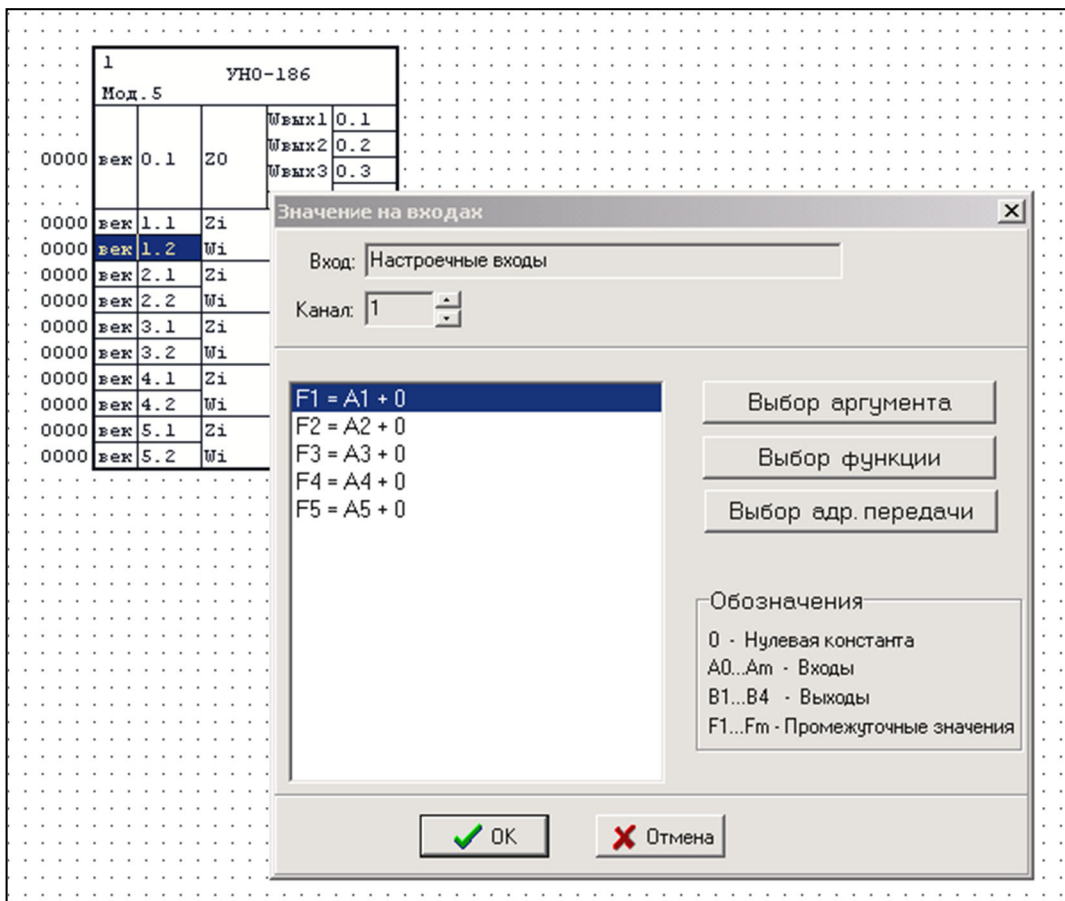
Рисунок 41 - Диалоговое окно программирования алгоритма УНО
