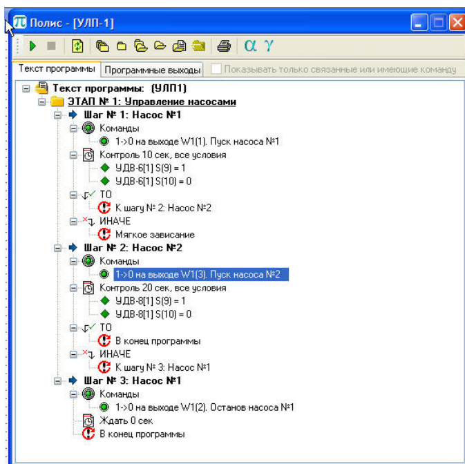
Рисунок 58 - Пример записи текста программы с условиями
