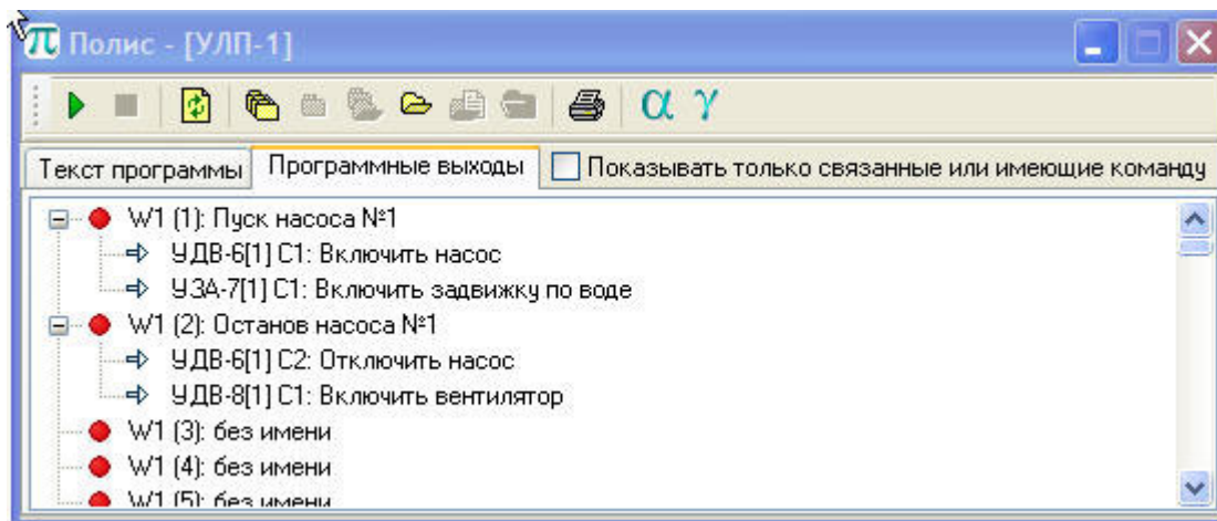
Рисунок 54 - Конфигурирование программных выходов (пример)
