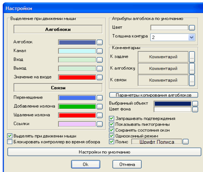
Рисунок 13 - Диалоговое окно настроек Пилона
