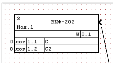
Рисунок 26 – Ссылка на выходе алгоблока
