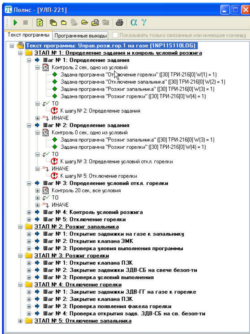
Рисунок 48 - Вид шаговой программы в окне закладки Текст программы (пример)
