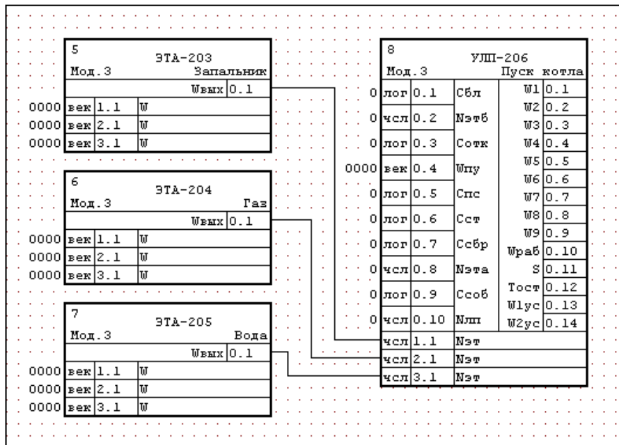
Рисунок 47 - Конфигурирование логической программы (пример)
