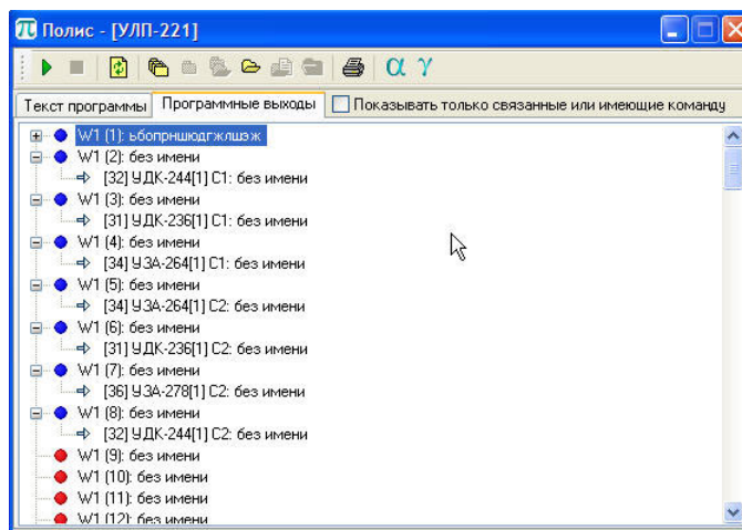
Рисунок 49 - Вид программы в окне закладки Программные выходы (пример)
