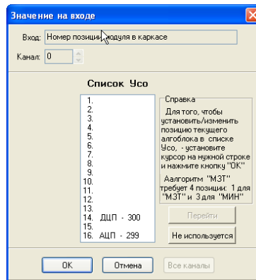
Рисунок 22 - Установка уникальной константы (пример 1)
