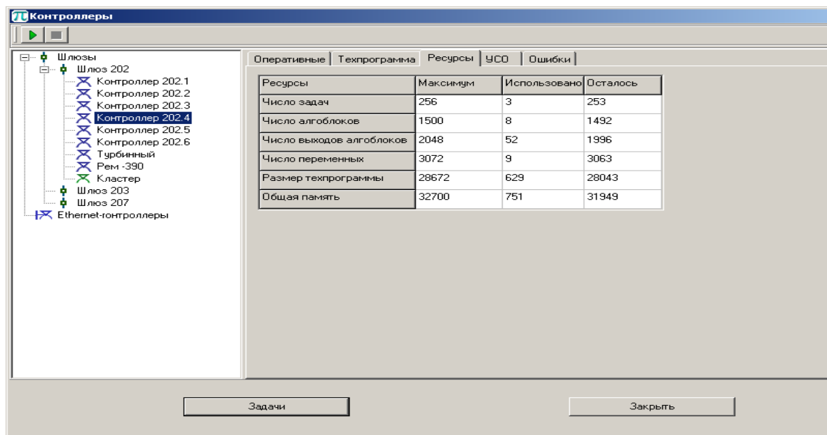
Рисунок 3 – Окно Контроллеры. Закладка Ресурсы
