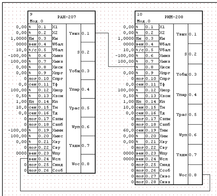
Рисунок 39 - Пример каскадного регулятора
