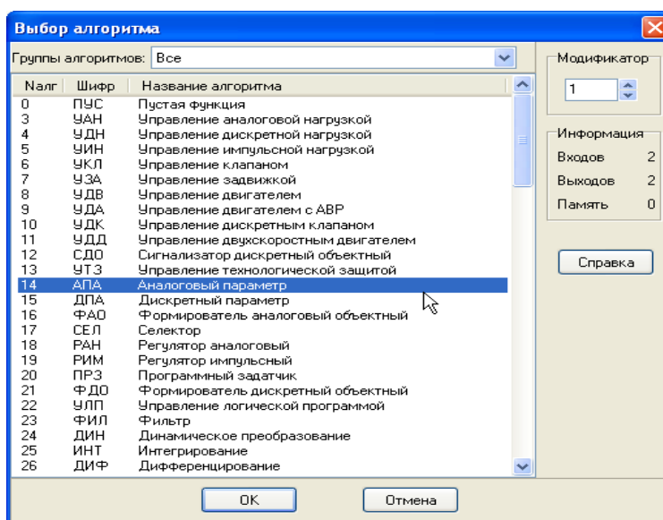
Рисунок 17 - Список библиотечных алгоритмов
